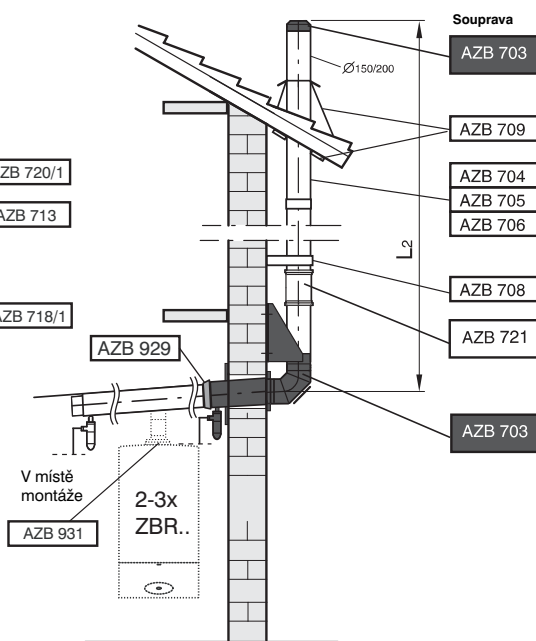
Odkouření na fasádu
