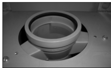
Připojovací místo pro odkouření u nových kondenzačních kotlů řad CERAPUR...
