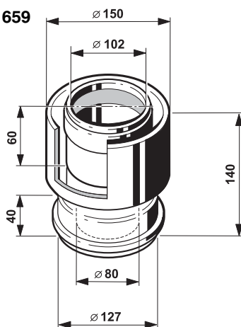
Použití AZB 659 v soupravě AZB 652/1
