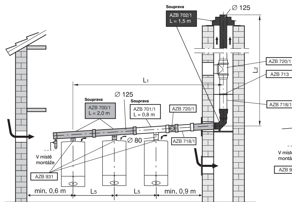
Odkouření komínem
